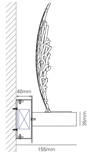
Zijaanzicht / Side view
